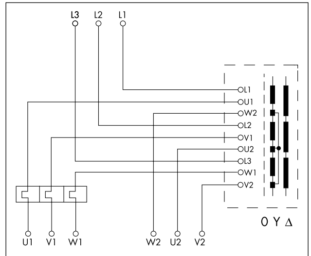
Stern-/Dreieckschalter KS mit Motorschutz, mit/ohne Unterspannungsauslösung 400 Volt (MS in Phase, jedoch Nennstrom einstellen)
