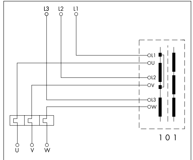
Wendschalter KW mit Motorschutz, mit/ohne Unterspannungsauslösung 400 Volt
