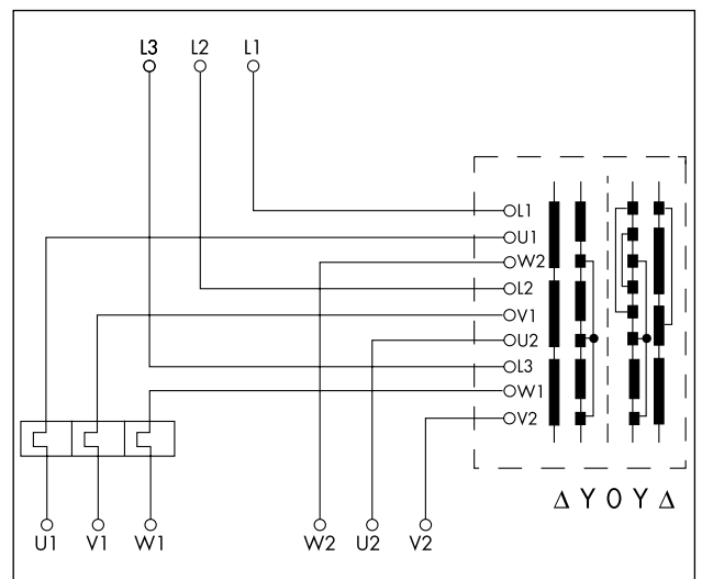
Stern-/Dreieckwendschalter KSW mit Motorschutz, mit/ohne Unterspannungsauslösung 400 Volt (MS in Phase, jedoch Nennstrom einstellen)
