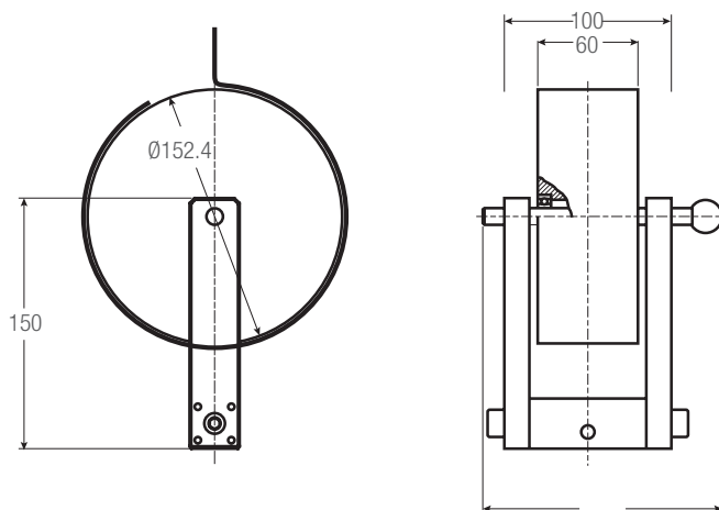
PEEL-3-D53357B-KL
